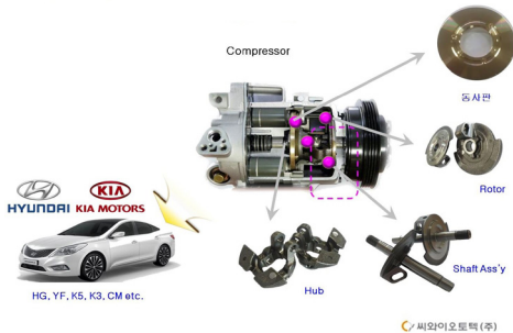
내연기관 승용차용 에어컨 컴프레서 구동 부품
