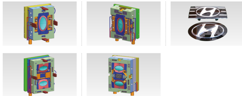
스팀 공법 + In Mold + 이중사출 적용한 SCC COVER 금형 제작
