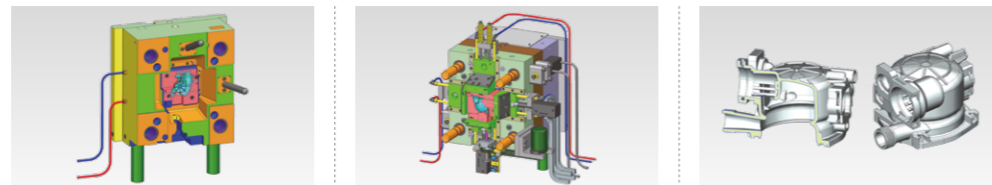
내측 언더컷 해결을 위해 탄성 코어 적용 금형 제작
